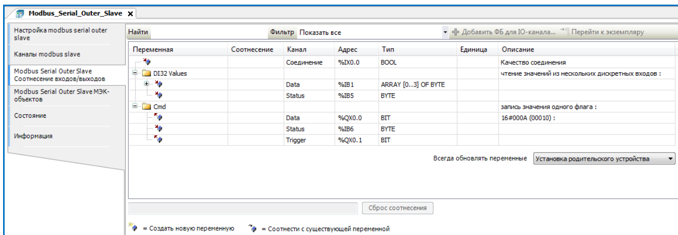
Рисунок 14 – Вкладка «Modbus Serial Outer Slave Соотнесение входов/выходов»
