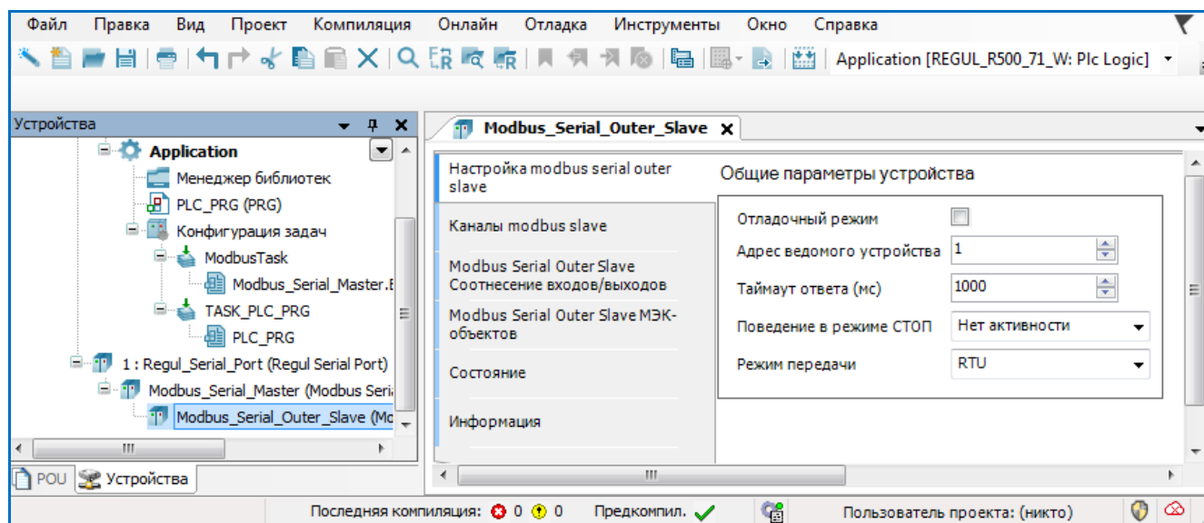
Рисунок 8 – Настройка параметров modbus serial outer slave
