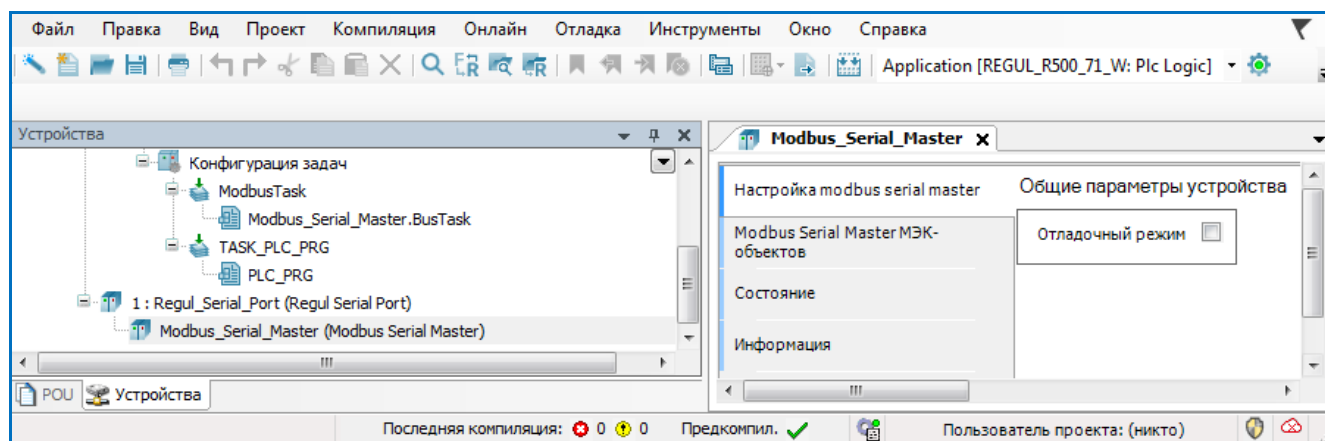
Рисунок 7 – Настройка параметров modbus serial master
