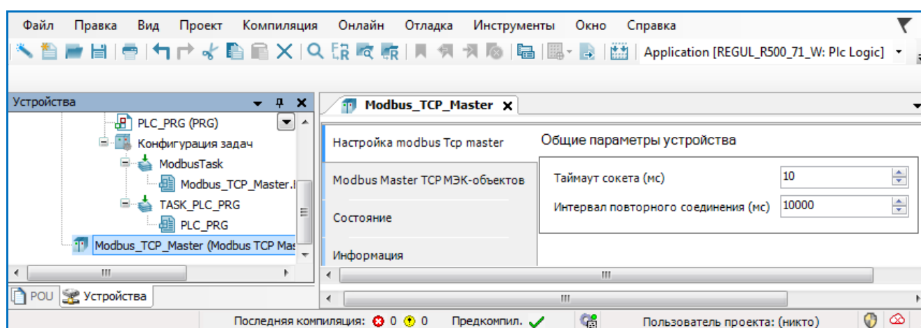
Рисунок 24 – Общие параметры Modbus TCP Master
