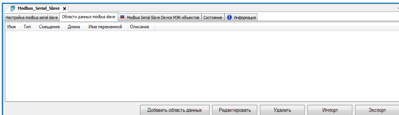
Рисунок 18 – Вкладка «Области данных Modbus slave»
