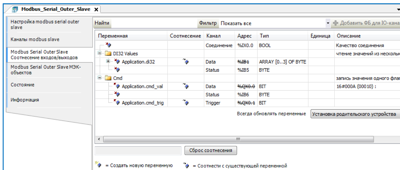
Рисунок 16 – Вкладка «Modbus Serial Outer Slave Соотнесение входов/выходов»
