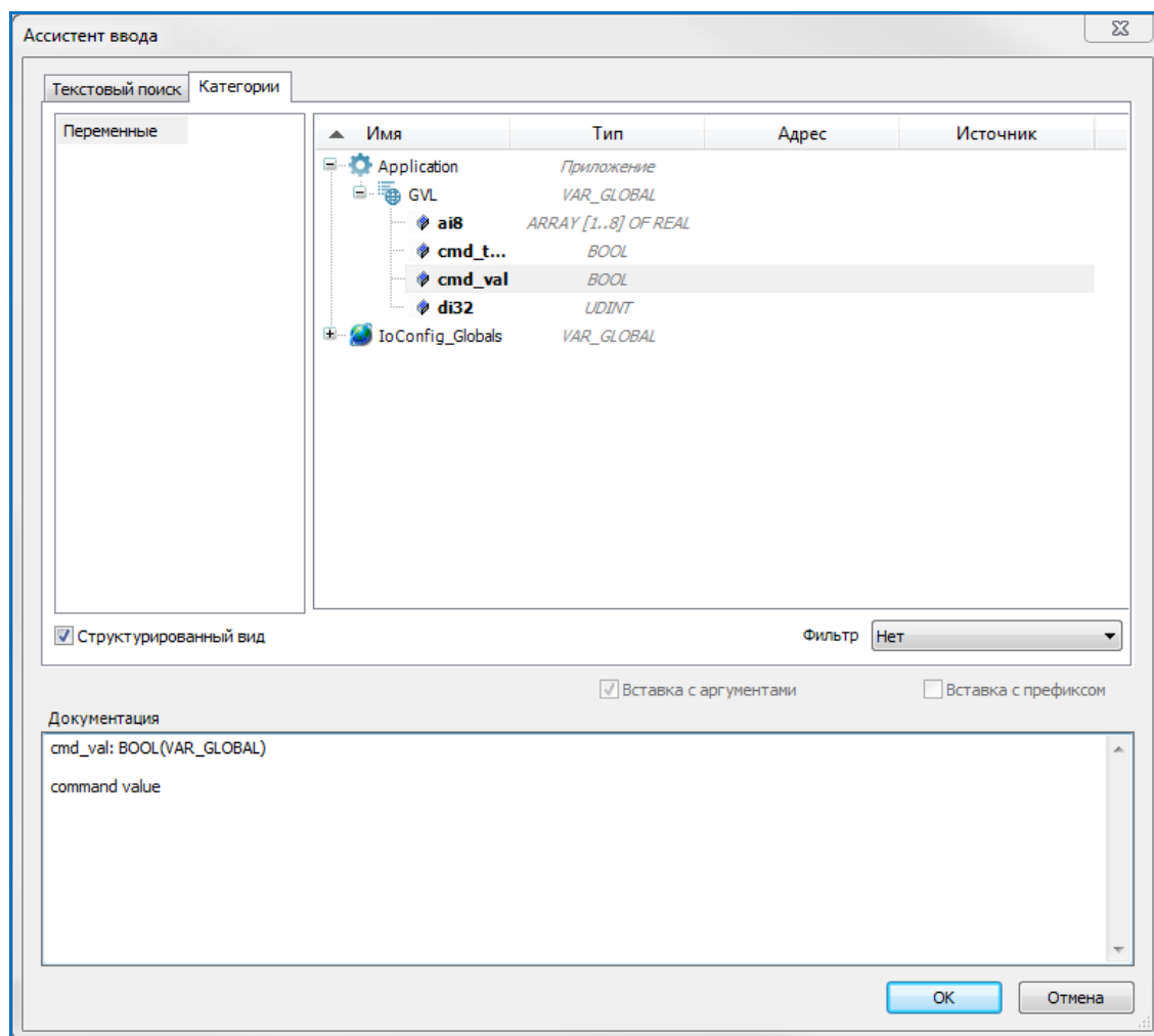
Рисунок 15 – Диалоговое окно «Ассистент ввода»
