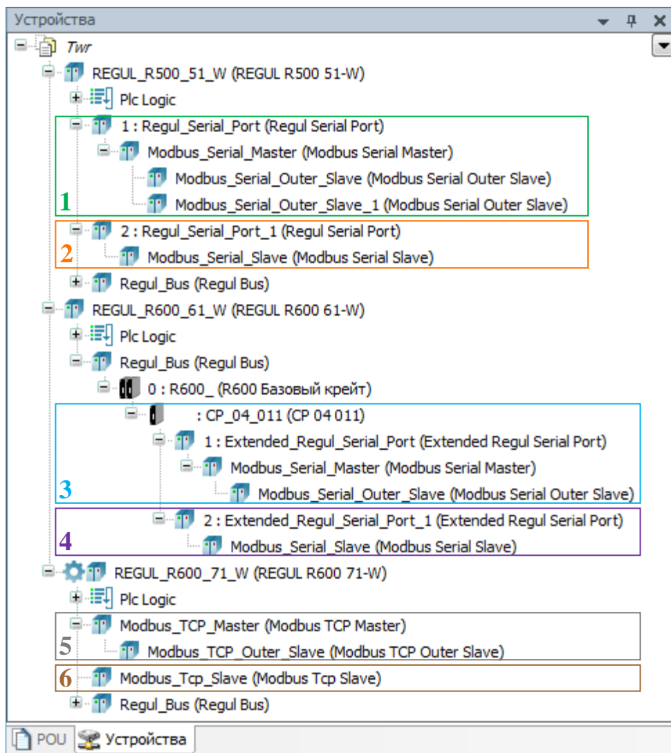
Рисунок 4 – Конфигурация устройств для различных режимов Modbus
