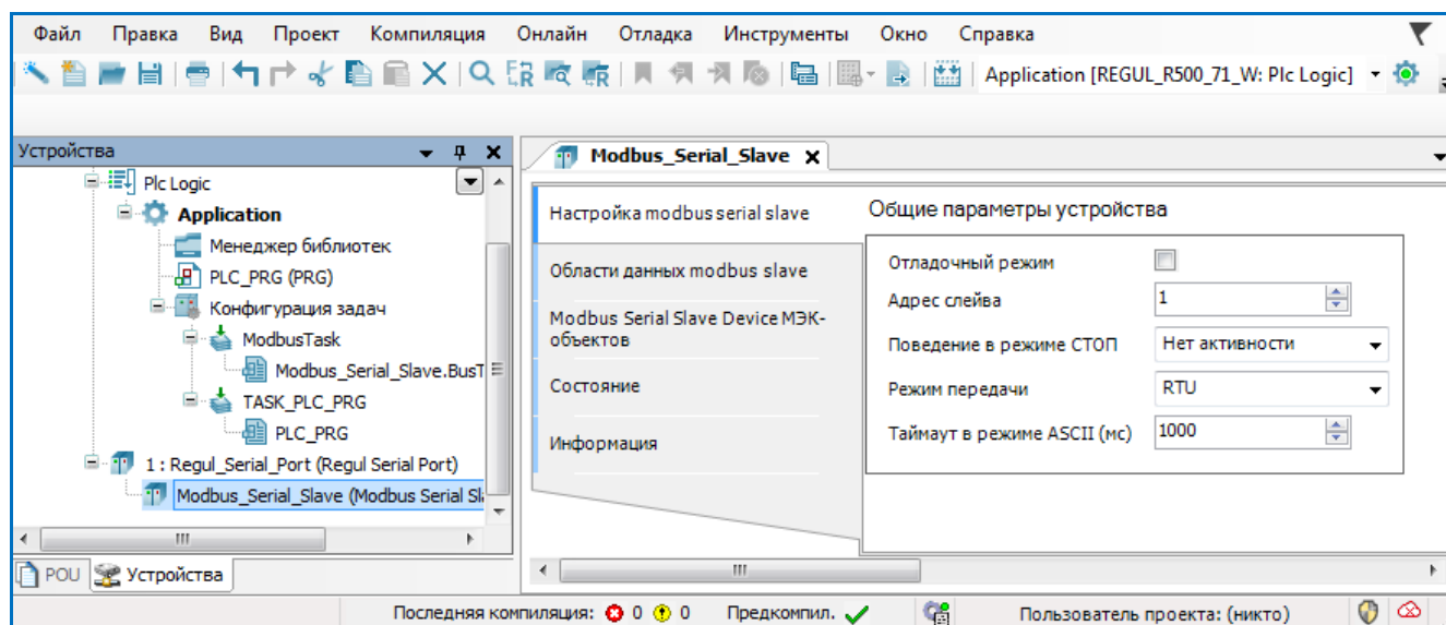
Рисунок 17 – Настройка параметров modbus serial slave
