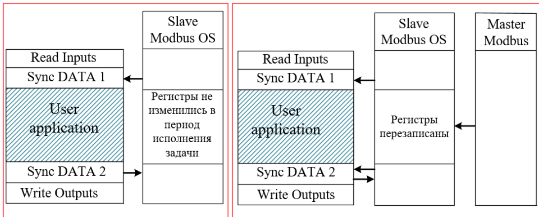
Рисунок 23 - Особенности работы драйвера Modbus Slave OS
