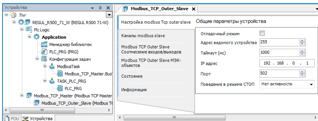
Рисунок 25 – Настройка параметров modbus Tcp outer slave
